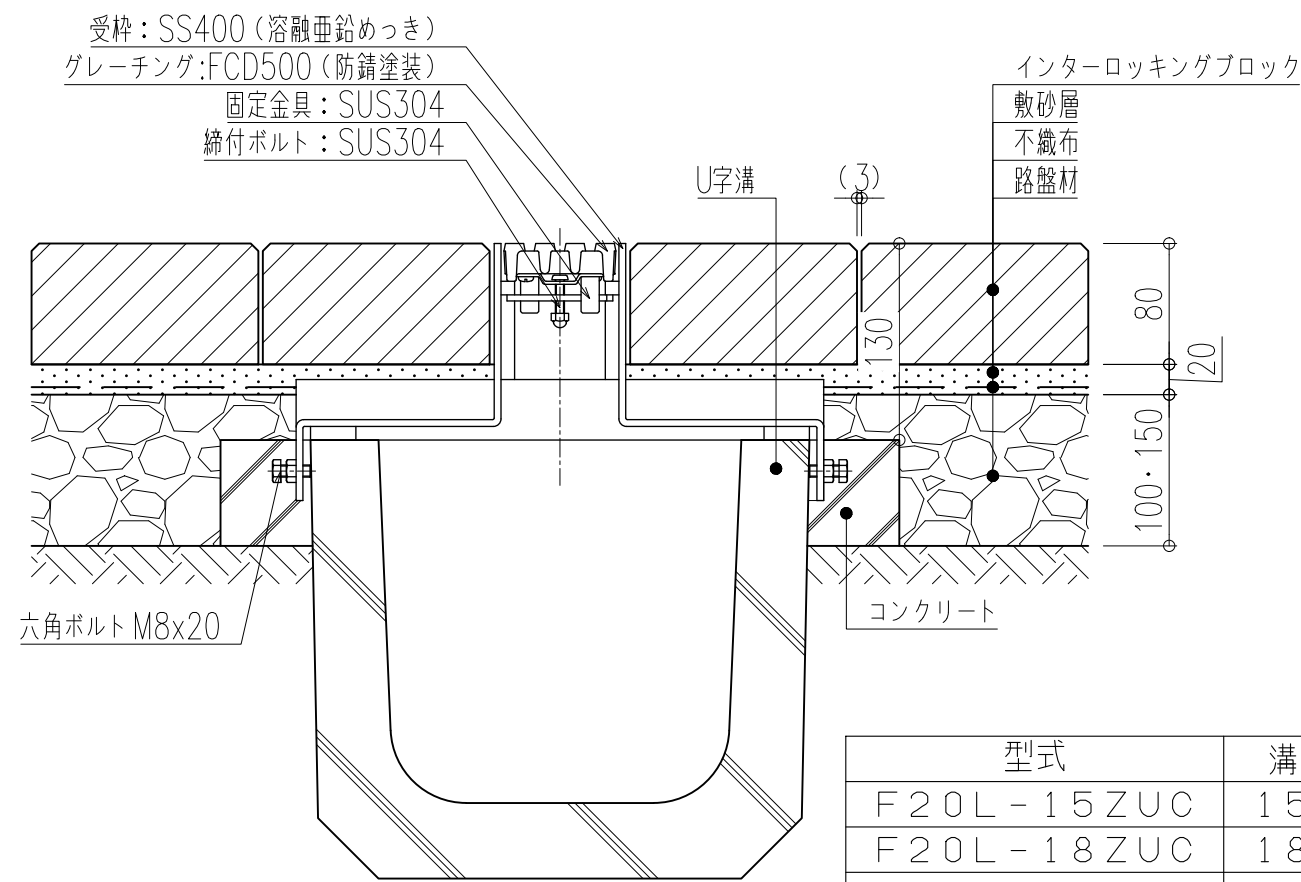
施工参考図
